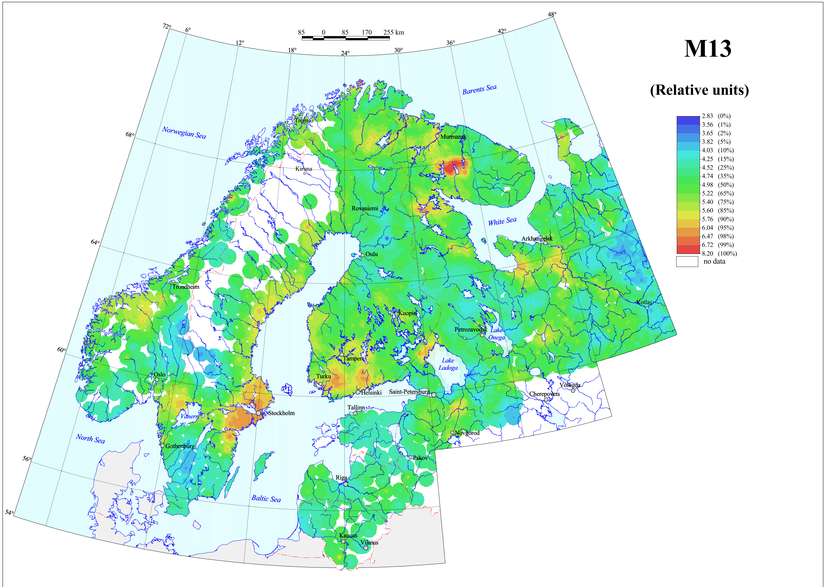
M13 (Na, K) in C-horizon, Grain Size <2 mm, Aqua regia Extraction
